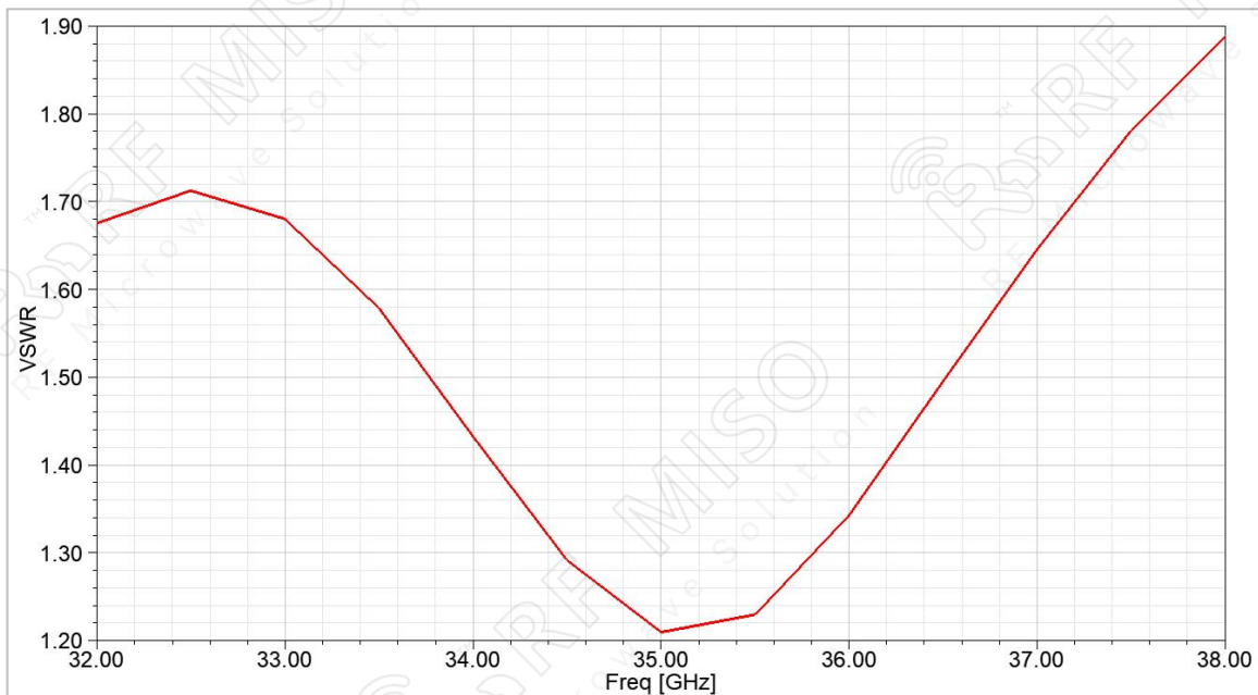
VSWR
