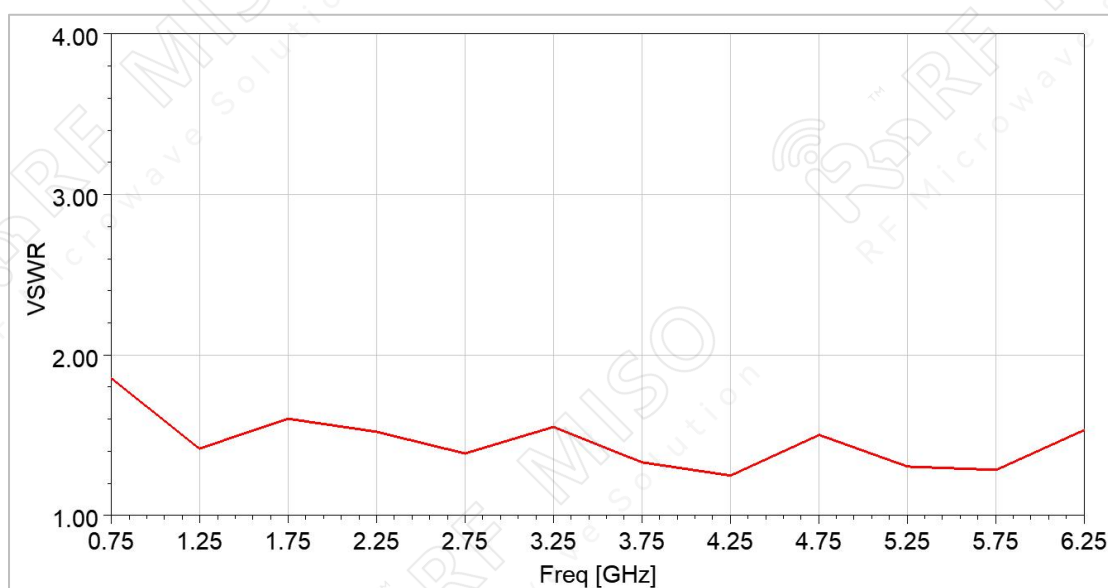
VSWR
