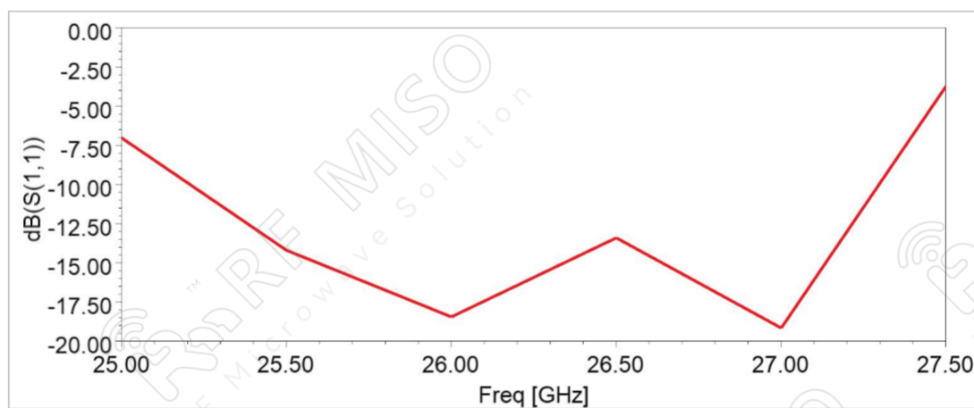
Return Loss(dB)
