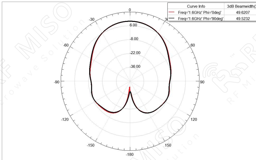
1.6 GHz
