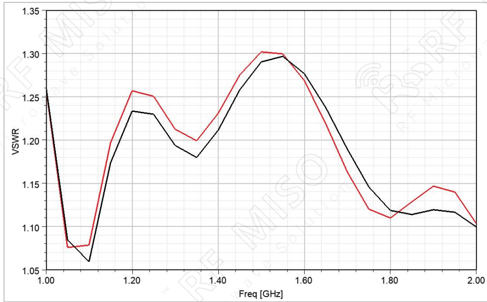
VSWR
