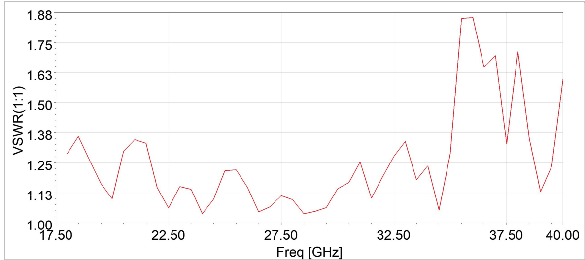
VSWR
