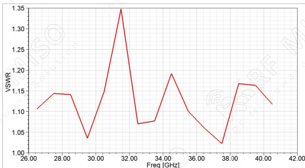
VSWR
