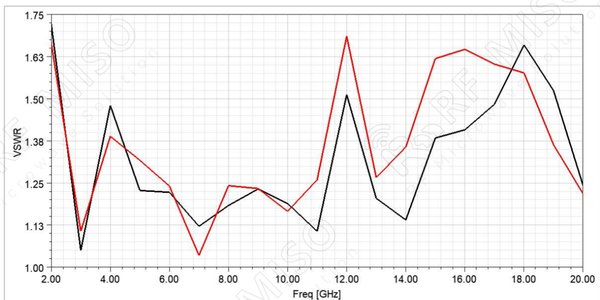
VSWR
