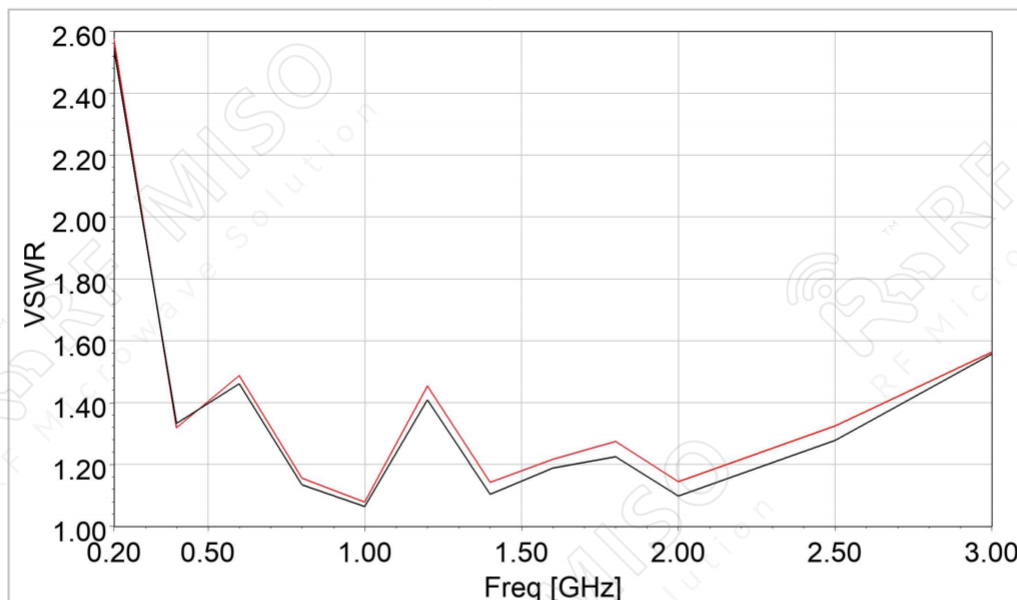
VSWR
