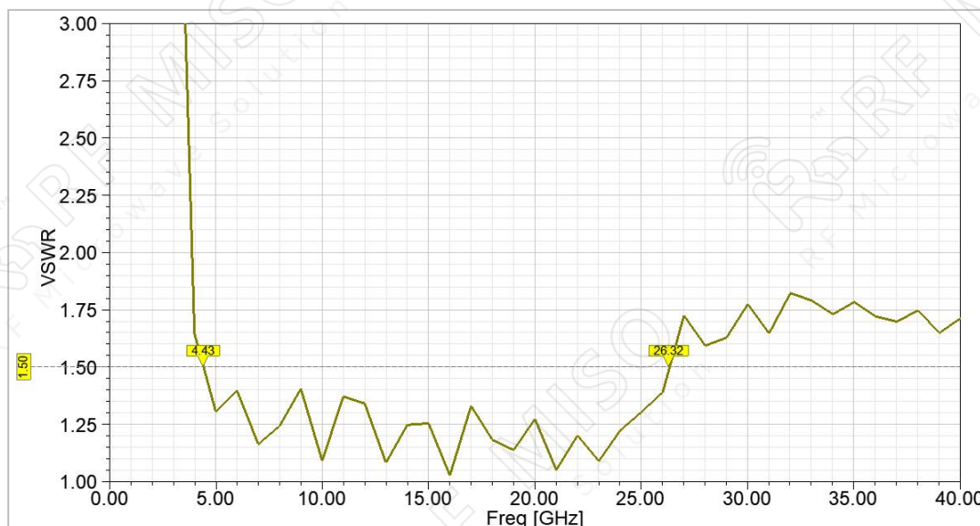
VSWR
